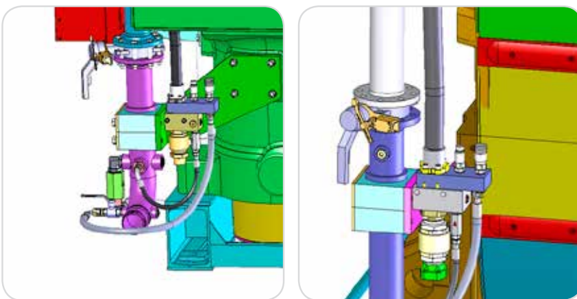
Rendering 3D del montaggio del kit di attacco rapido
